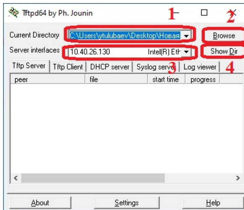
Рис. 1: Окно Tftpd64
